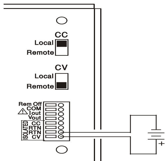
Konstantstromsteuerung
