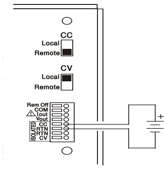
Comando tensione costante
