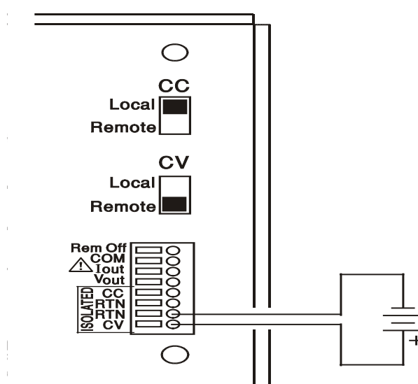
Comando corrente costante
